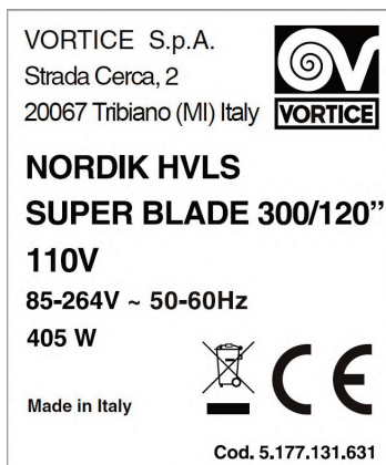
Fig. 1 - exemple plaque signalétique pour SUPER BLADE 300/120" 110V
